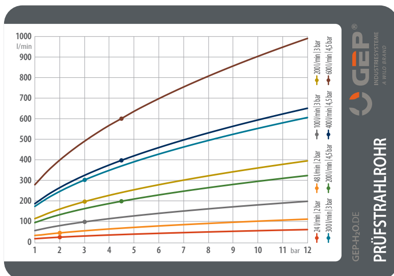
Einleger Prüfstrahlrohr (vergrößerte Darstellung).
