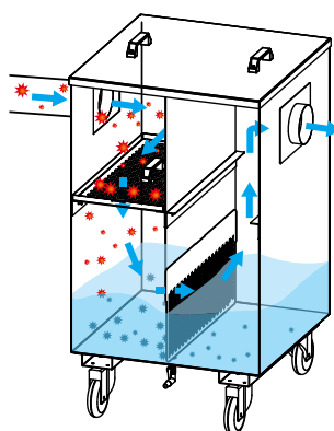
Wasserbadvorabscheider
