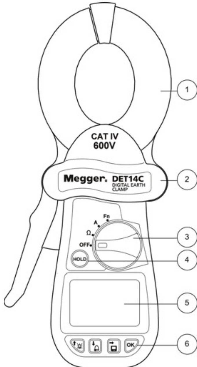
Abbildung 1: DET14C / DET24C Vorderansicht
