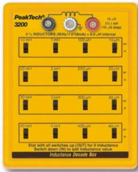
PeakTech® 3200 Induktivitätsdekade
