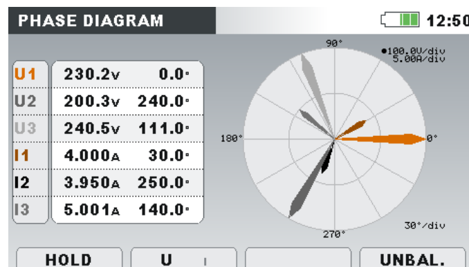
Abbildung 3.36: Bildschirm des Phasendiagramms
