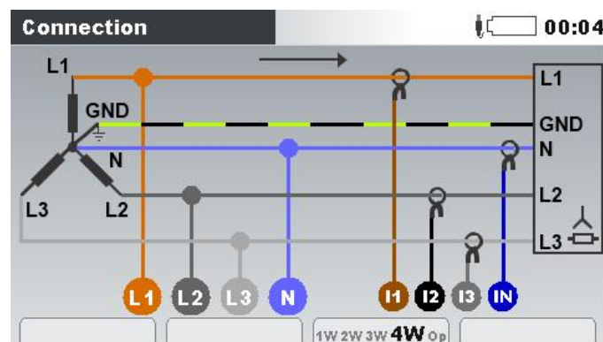
Abbildung 4.3: Auswählen des dreiphasigen 4-Leitersystem auf dem Gerät
