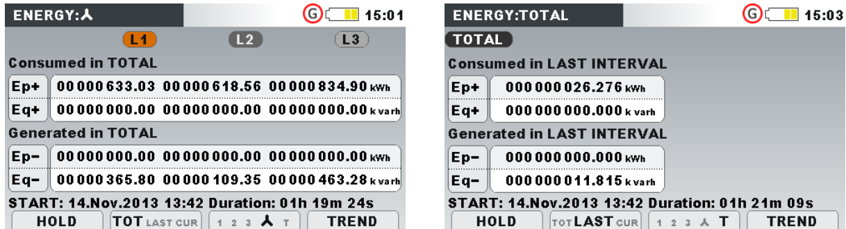
Abbildung 3.27: Bildschirm mit den Energiezählern
