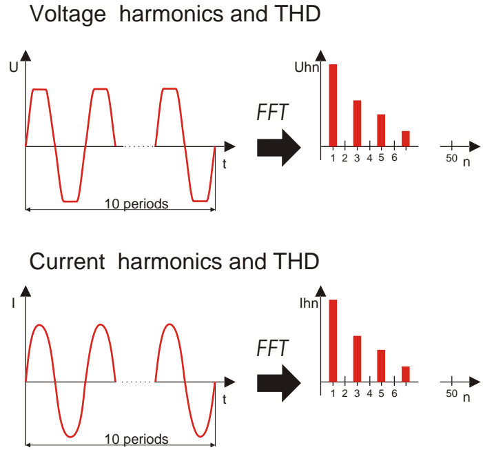
Abbildung 5.6: Strom- und Spannungsharmonische
