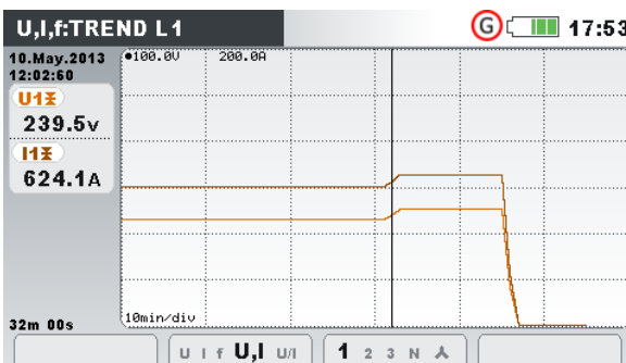
Abbildung 3.18: Spannungs- und Stromtrend (Einfach-Modus)
