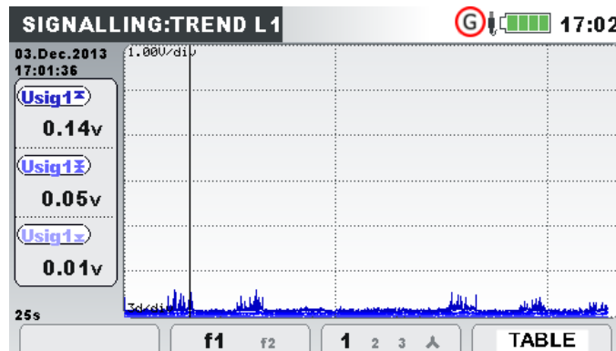
Abbildung 3.44: Bildschirm mit dem Trend der Netzsignale
