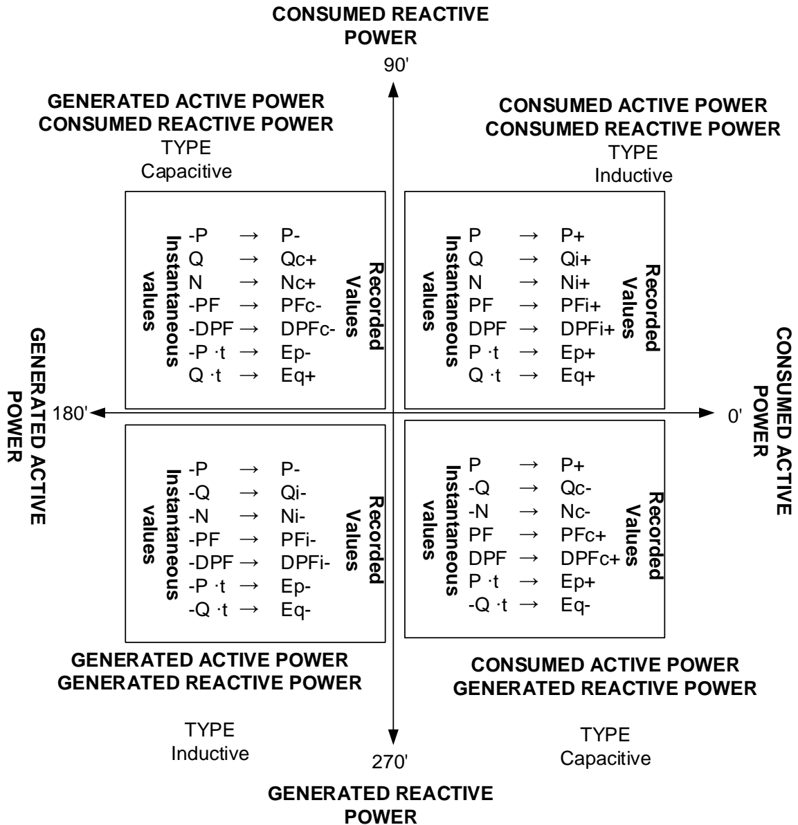
Abbildung 5.15: Phasen-/Polaritätsdiagramm zu Verbrauch/Erzeugt und Induktiv/Kapazitiv
