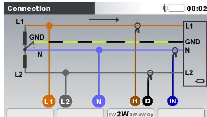
Abbildung 4.11: Auswählen des zweiphasigen 4-Leitersystem auf dem Gerät
