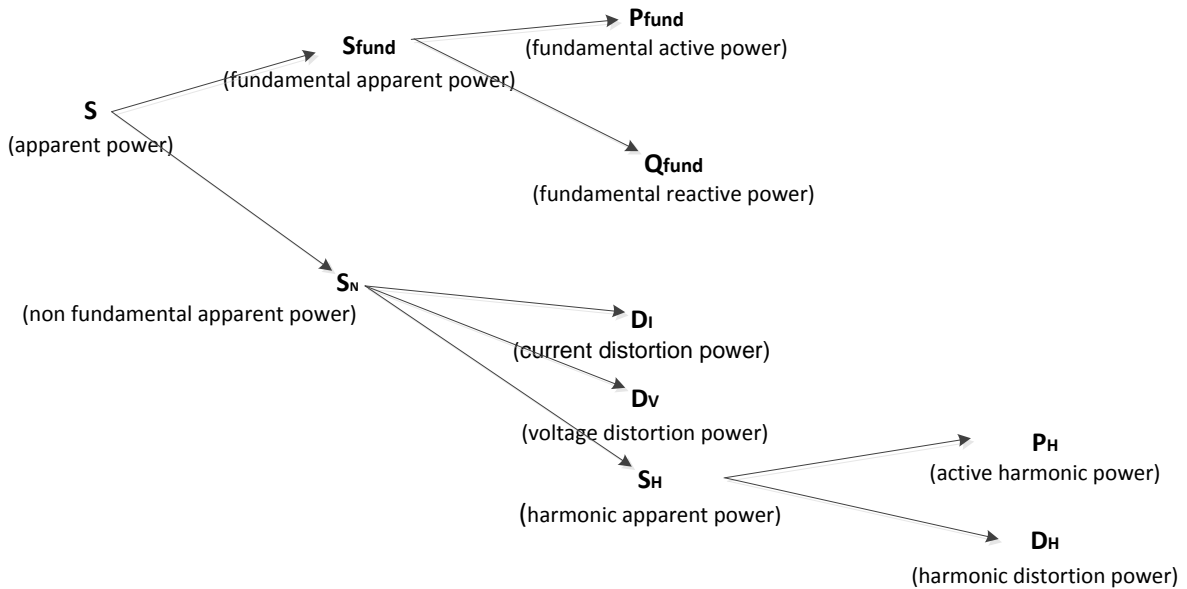
Abbildung 5.2: IEEE 1459 Organisation der Phasenleistungsmessung (Phase)
