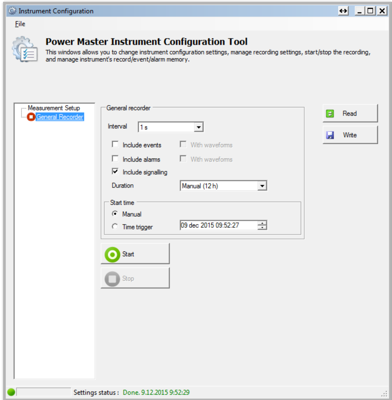
Abbildung 4.27: Formular zur Konfiguration des Remote-Geräts
