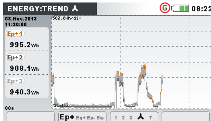
Abbildung 3.28: Bildschirm Energietrend
